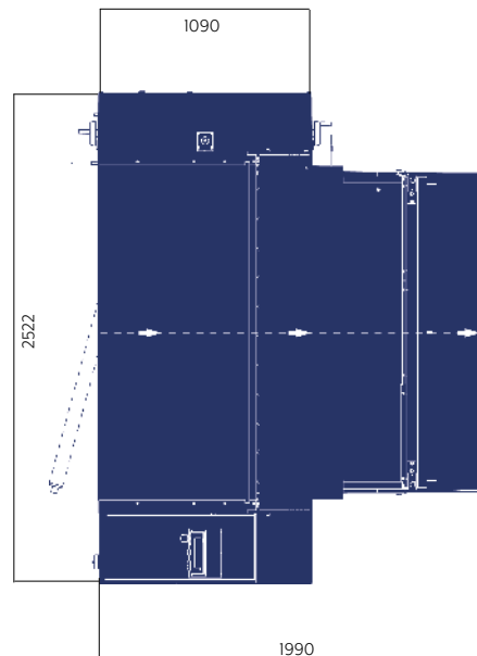
Floorplan KS 601
